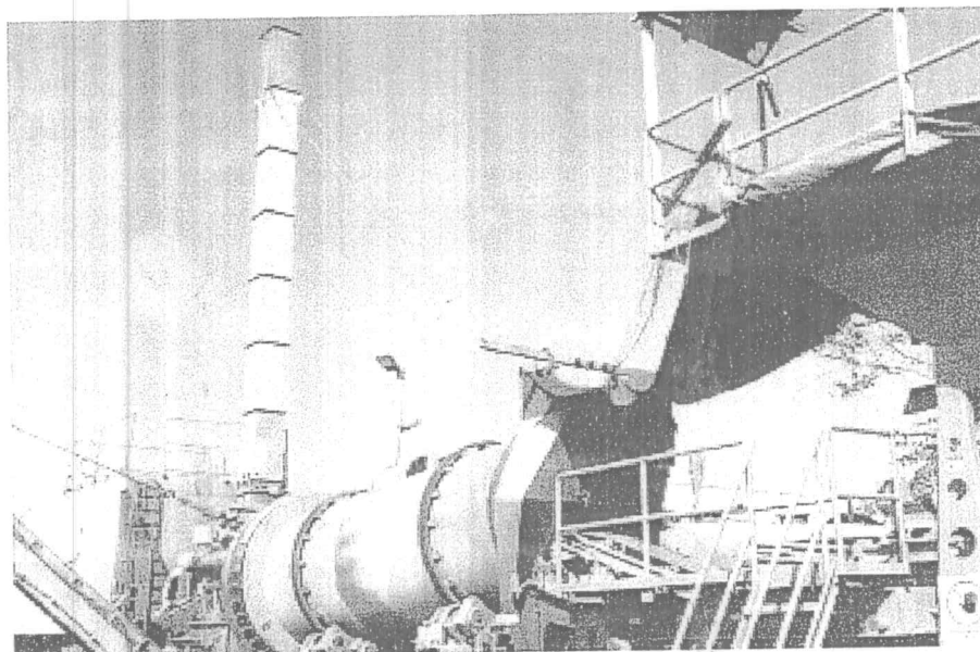
Figura 2. Sistema secado y quemador.
